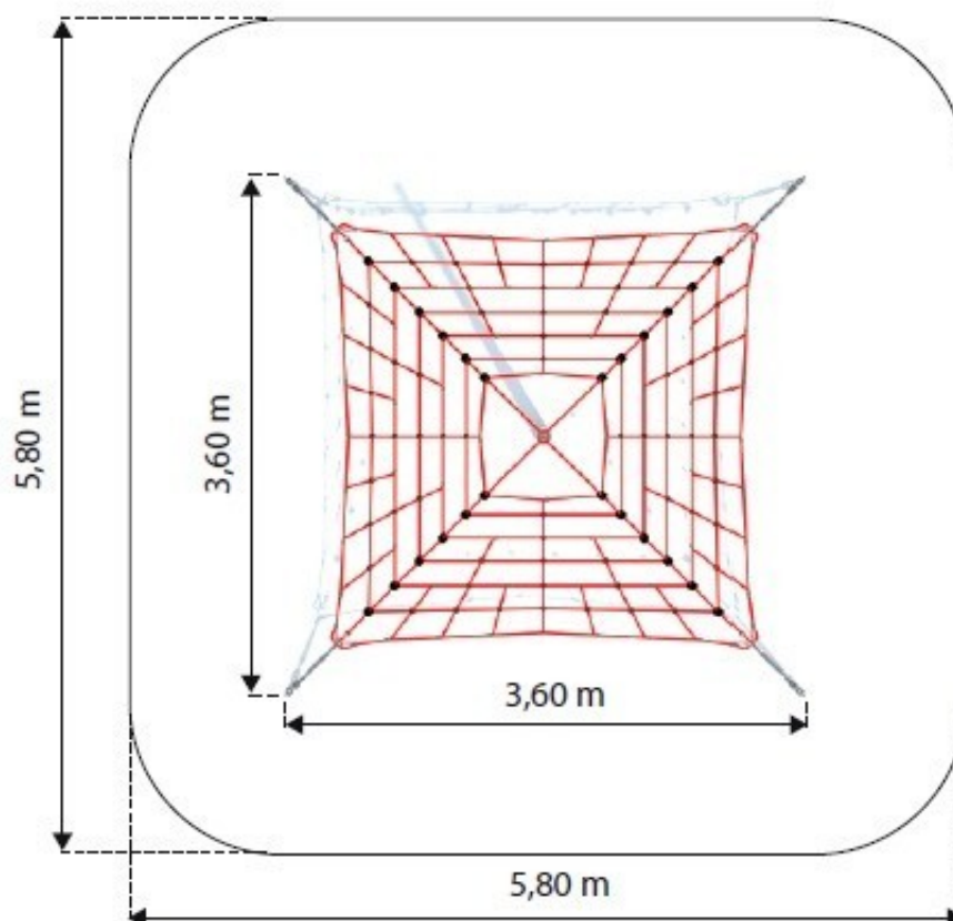
Zał. 1. Wymiary urządzenia i strefy bezpieczeństwa
